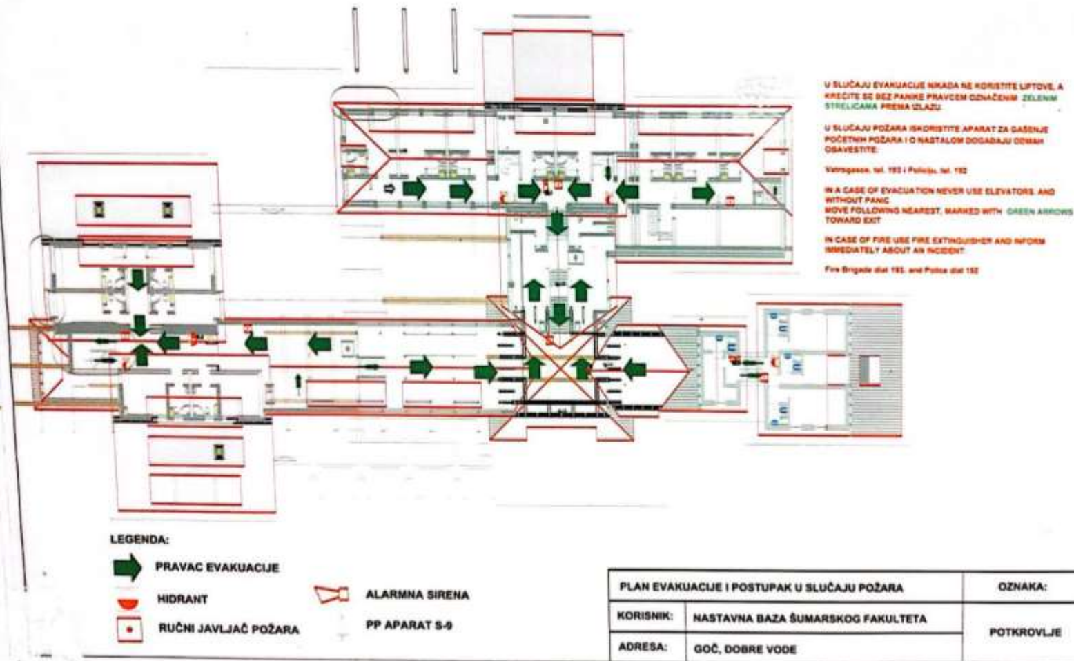
Слика 18. План евакуације - Наставна база „Гоч“ - основа поткровља
