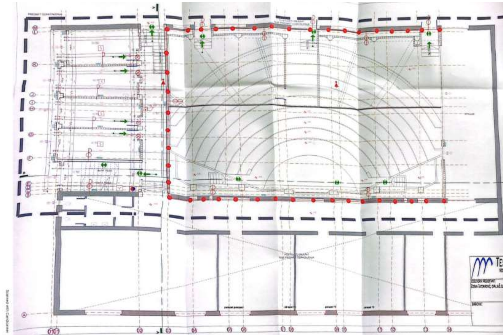
Слика 14. План евакуације - Шумарски факултет - основа првог спрата
