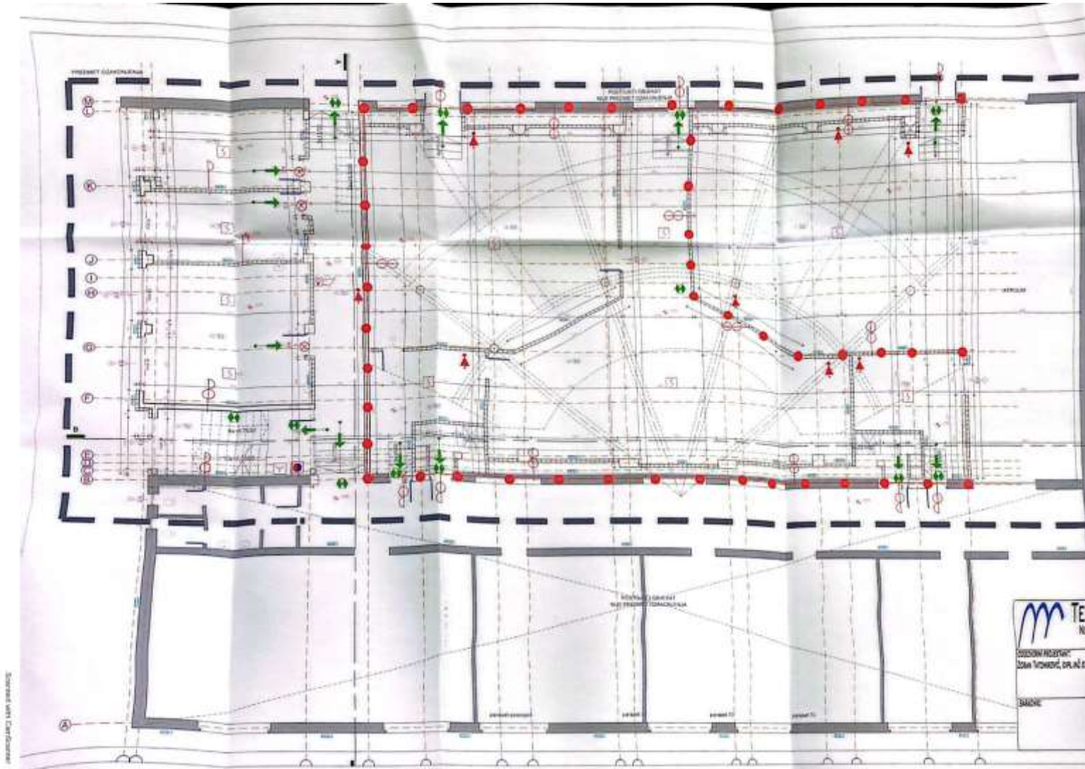
Слика 13. План евакуације - Шумарски факултет - основа приземља
