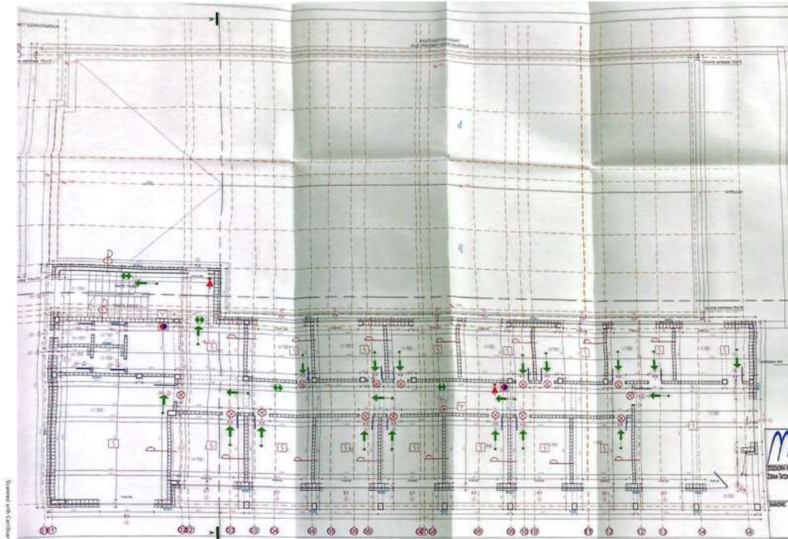
Слика 16. План евакуације - Шумарски факултет - основа трећег спрата
